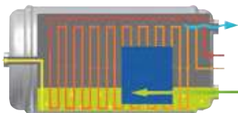
SISTEMA DI DISTILLAZIONE INTEGRATO
